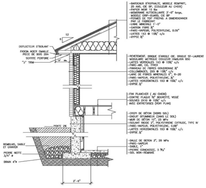
Coupe de mur
